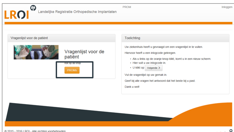
Afbeelding 1. Inlogpagina PROMs
